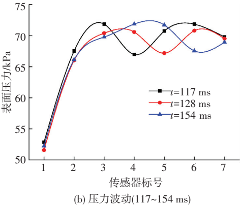
图 14 空泡脱落过程中航行体表面压力
