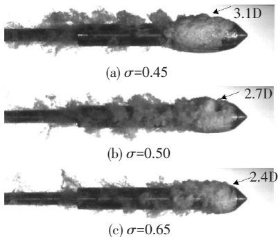
图 8 空泡脱落位置
