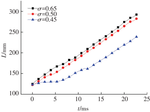
图 9 脱落空泡团的运动位移随时间的变化
