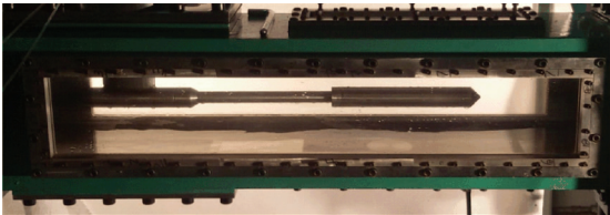
图 2 水洞工作段
