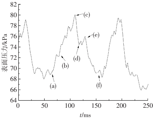
图 12 传感器 T_3 压力曲线
