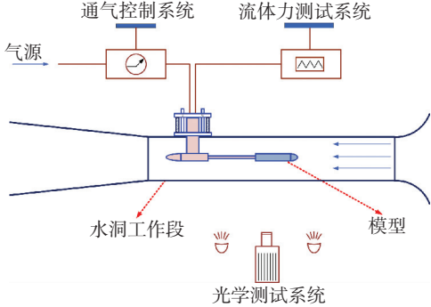
图 3 水洞实验系统示意
