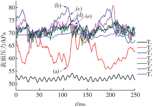
图 11 不同传感器的压力
