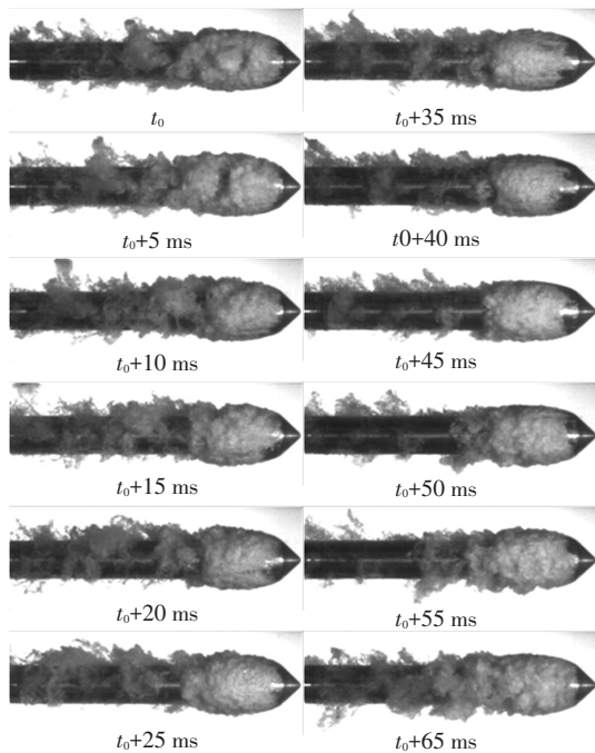
图 6 空泡脱落过程 ( \sigma=0.50 )
