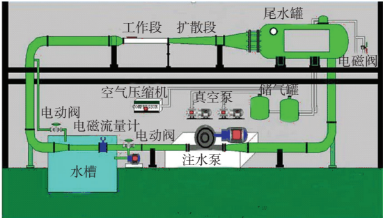
图 1 水洞示意
