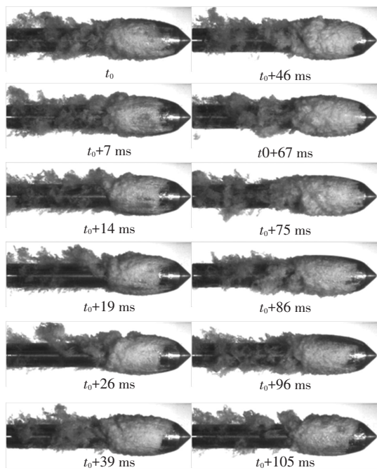
图 5 空泡脱落过程 ( \sigma=0.45 )
