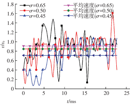
图 10 脱落空泡团运动的瞬时速度及平均速度
