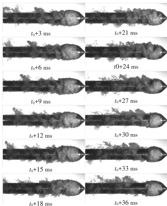
图 7 空泡脱落过程 ( \sigma=0.65 )
