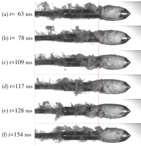
图 13 工况三空泡脱落
